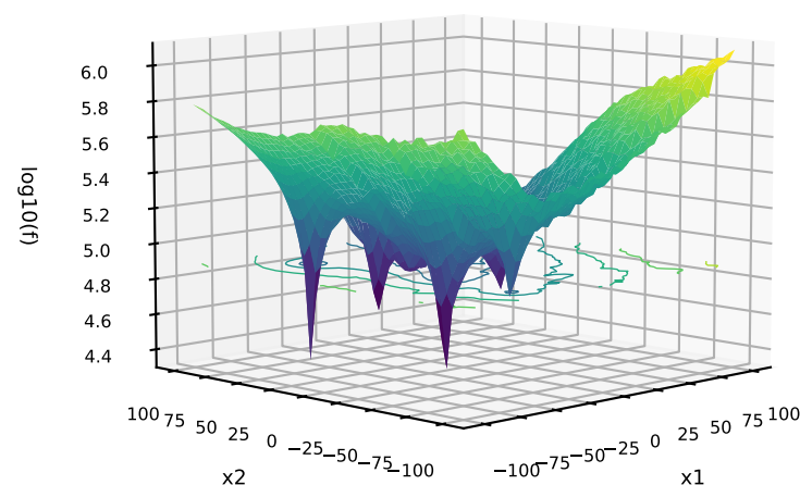
230: C=DPM-SOFTMAX; P=MIXED; T=MIXED G=StyblinskiTang+BentCigar Levy+SchafferF7+Rosenbrock
