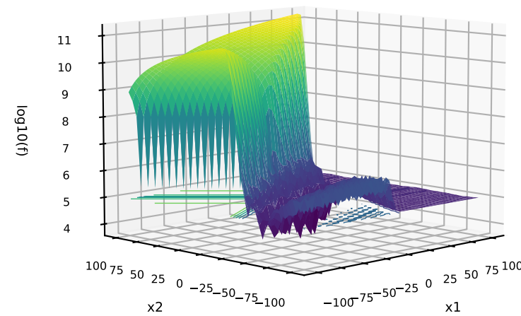
79: C=CPM-PMEAN; P=MIXED; T=MIXED G=Gallagher21+Schwefel+StyblinskiTang+Exponential Rosenbrock+Ackley+LunacekBIRastrigin+SchafferF6
