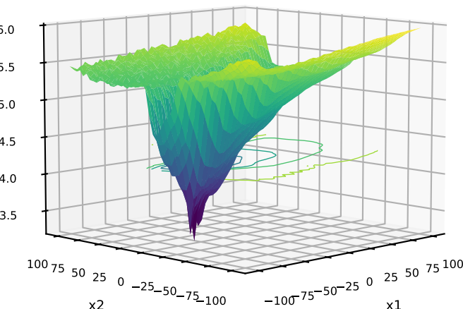
392: C=CPM-LWELL; P=MIXED; T=AF G=GriewankRosenbrock SchafferF6
