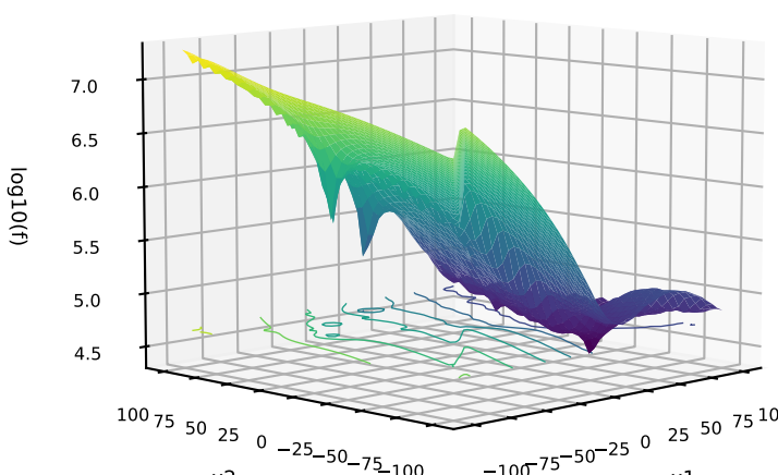
399: C=DPM-BGSOFTMAX; P=POWER; T=MIXED G=Katsuura+SchafferF7Cond1000 Rosenbrock
