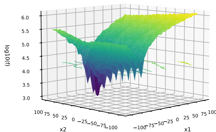
67: C=DPM-SOFTMAX; P=NONE; T=MIXED G=Griewank Griewank
