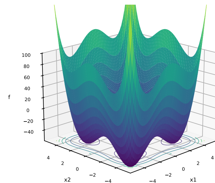
33: StyblinskiTang
