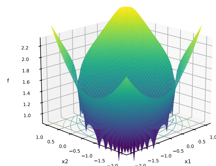
30: Step
