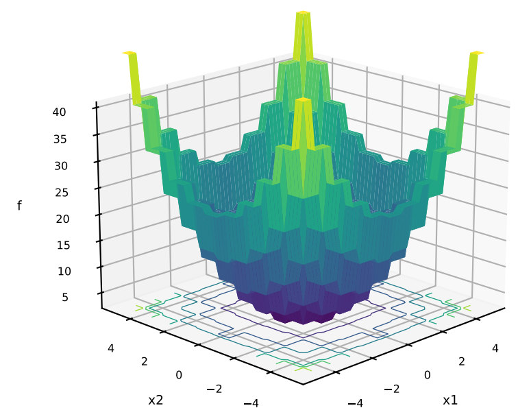
30: Step
