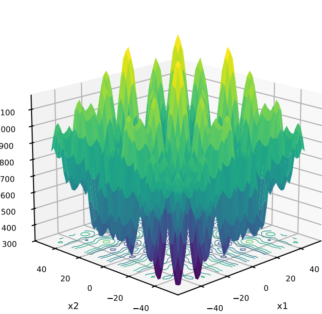
12: Schwefel
